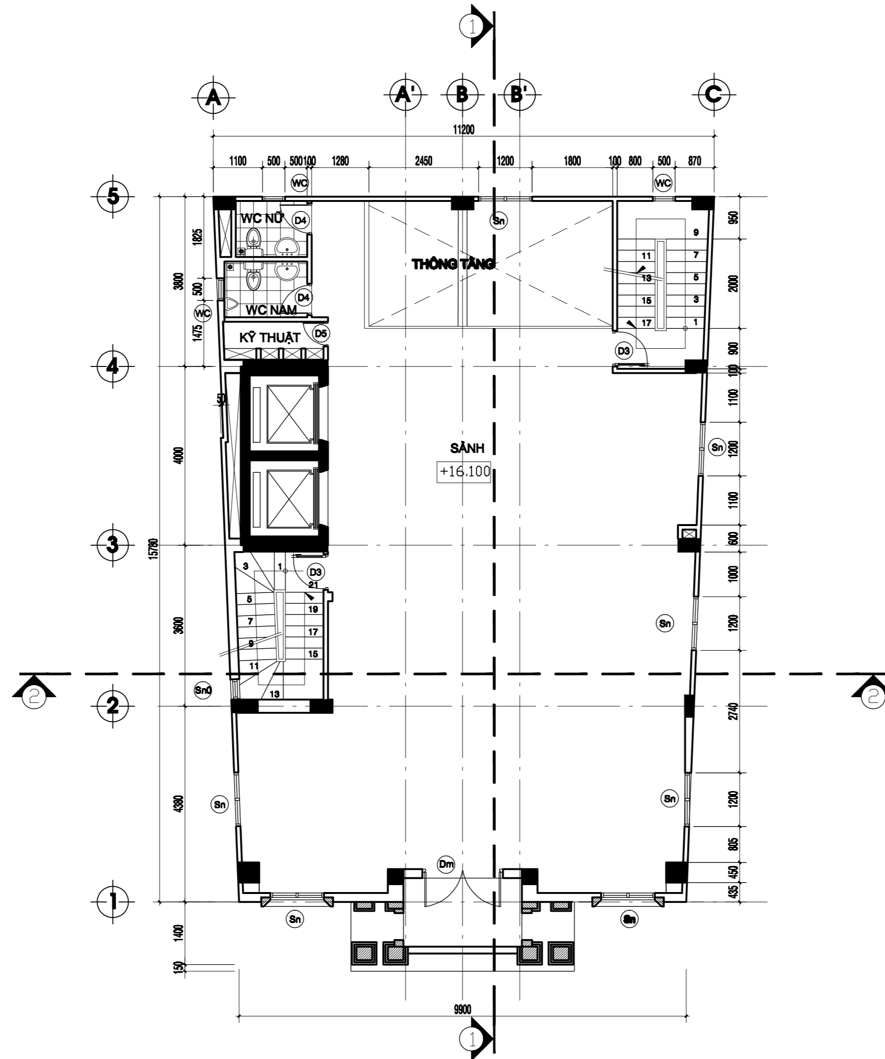
MẶT BẰNG LẦU 4 _ TL 1/100
