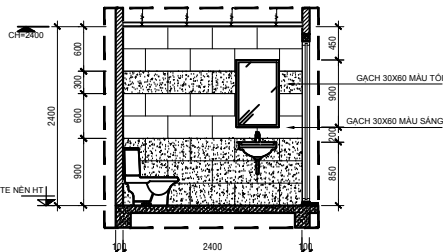
MẶT CẮT 2-2
