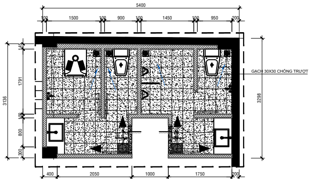
MẶT BẰNG LÁT GẠCH
