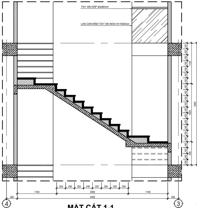
MẶT CẮT 1-1
