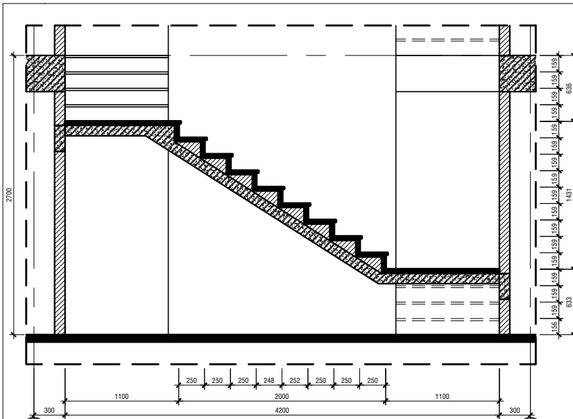
MẶT CẮT 1-1 TL: 1/25
