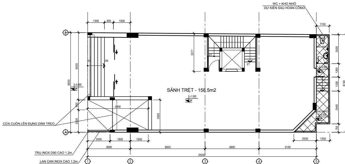
MẶT BẰNG TẦNG TRỆT TL: 1/100
