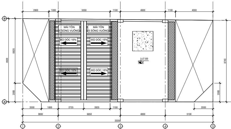
MẶT BẰNG MÁI TL: 1/100
