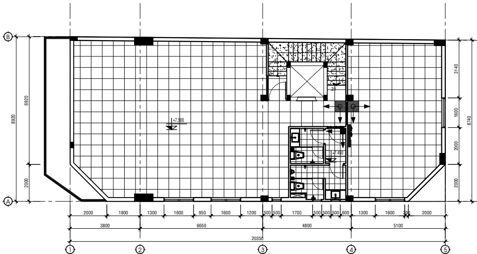
MẶT BẰNG LÁT GẠCH LẦU 1 TL: 1/100
