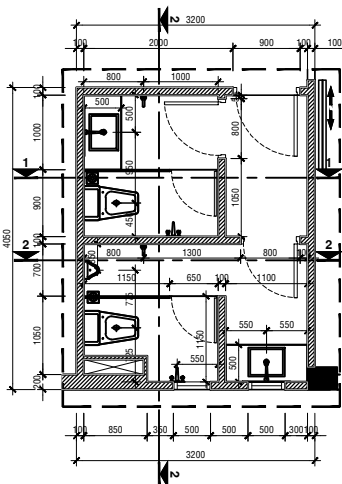
MẶT BẰNG KÍCH THƯỚC
