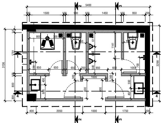
MẶT BẰNG KÍCH THƯỚC
