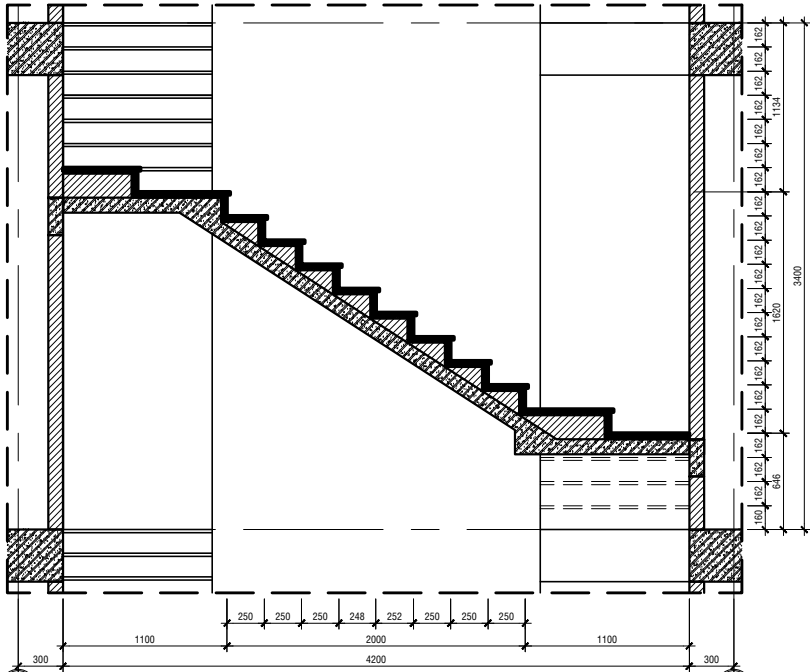
MẶT CẮT 1-1 TL: 1/25
