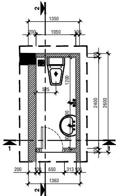
MẶT BẰNG KÍCH THƯỚC
