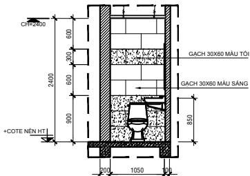
MẶT CẮT 1-1
