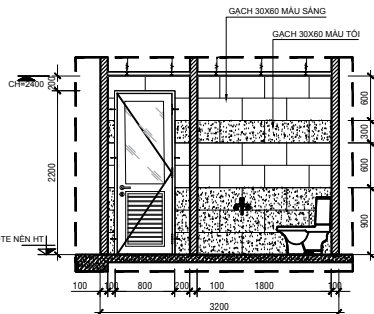
MẶT CẮT 1-1
