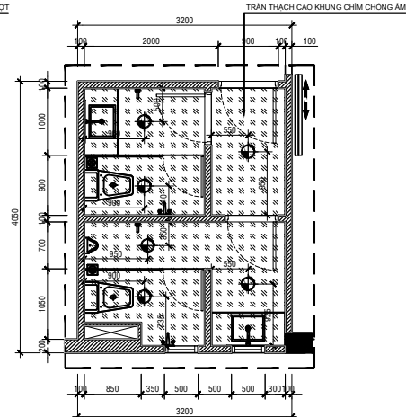
MẶT BẰNG TRẦN ĐÈN
