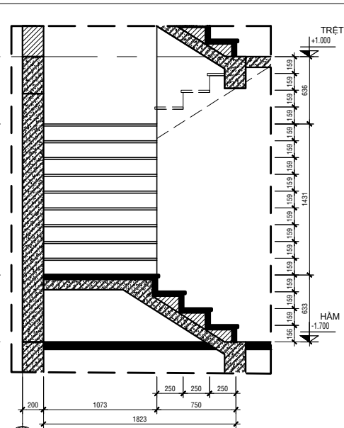
MẶT CẮT 2-2 TL: 1/25
