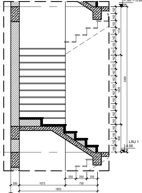
MẶT CẮT 2-2 TL: 1/25
