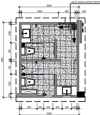
MẶT BẰNG LÁT GẠCH
