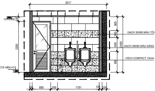
MẶT CẮT 3-3 TL: 1/50
