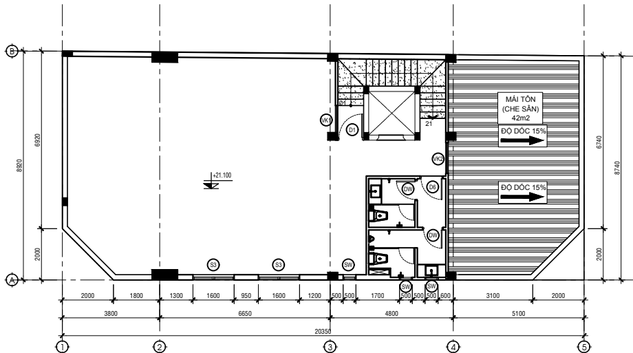
MẶT BẰNG ĐỊNH VỊ CỬA LẦU 5 TL: 1/100
