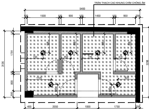
MẶT BẰNG TRẦN ĐÈN
