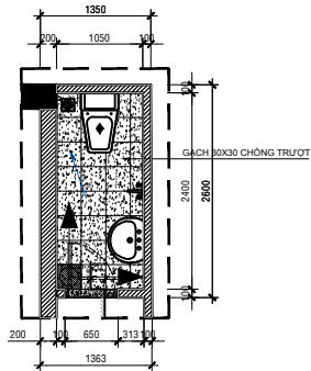
MẶT BẰNG LÁT GẠCH
