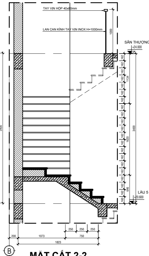
MẶT CẮT 2-2
