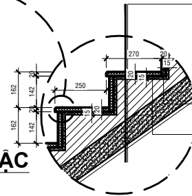
MẶT CẮT 2-2 TL: 1/25
