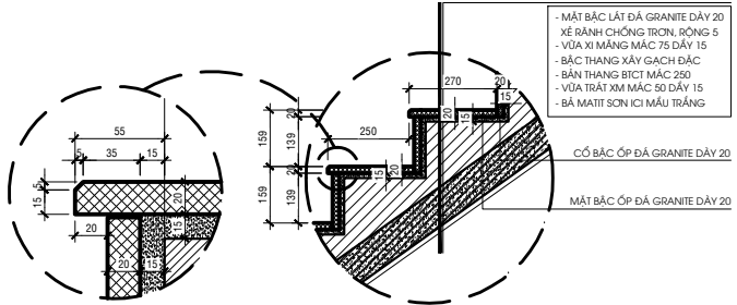
CHI TIẾT MŨI BẠC TL: 1/10
