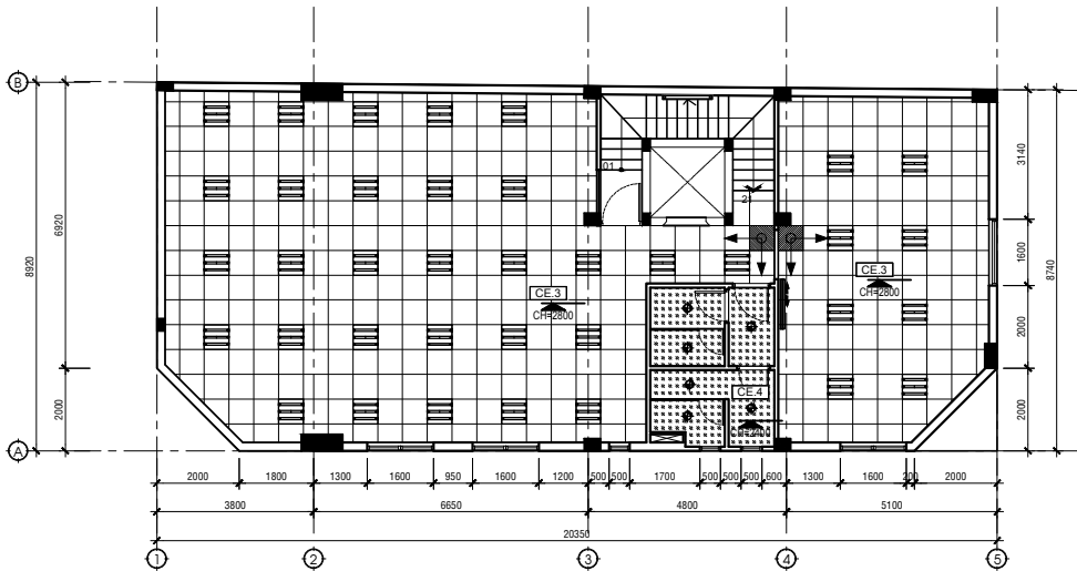
MẶT BẰNG TRẦN ĐÈN LẦU 1 TL: 1/100
