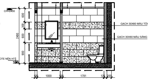
MẶT CẮT 2-2 TL: 1/50
