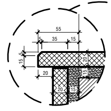
CHI TIẾT MŨI BẠC TL: 1/10
