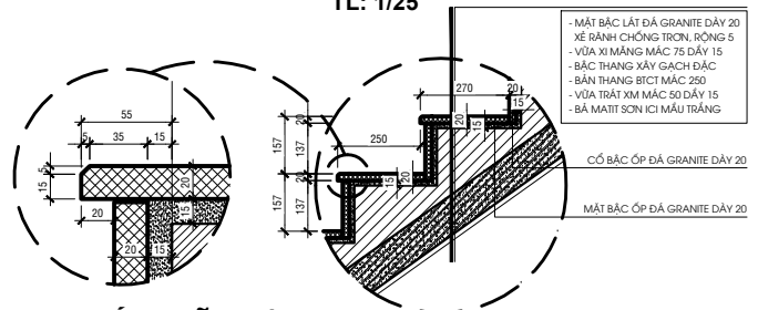
CHI TIẾT MŨI BẠC TL: 1/10
