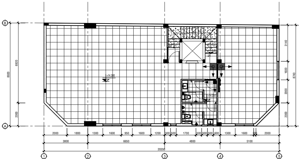
MẶT BẰNG LÁT GẠCH LẦU 3 TL: 1/100
