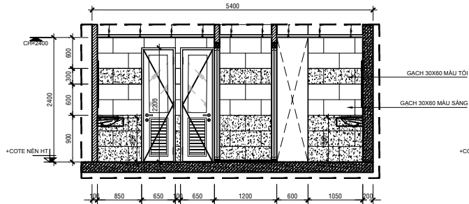
MẶT CẮT 4-4 TL: 1/50
