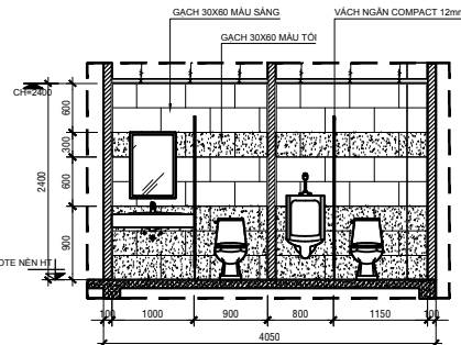
MẶT CẮT 3-3
