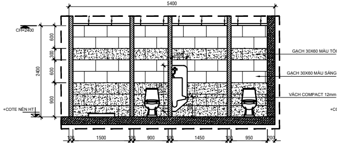
MẶT CẮT 1-1 TL: 1/50
