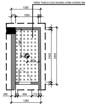
MẶT BẰNG TRẦN ĐÈN
