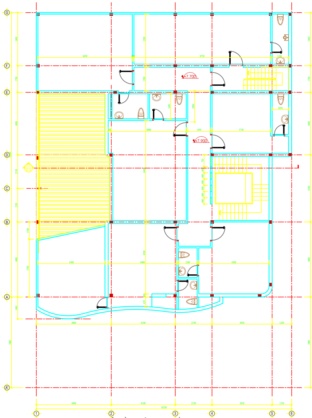
MẶT BẰNG HIỆN TRẠNG LẦU 2 TL: 1/100
