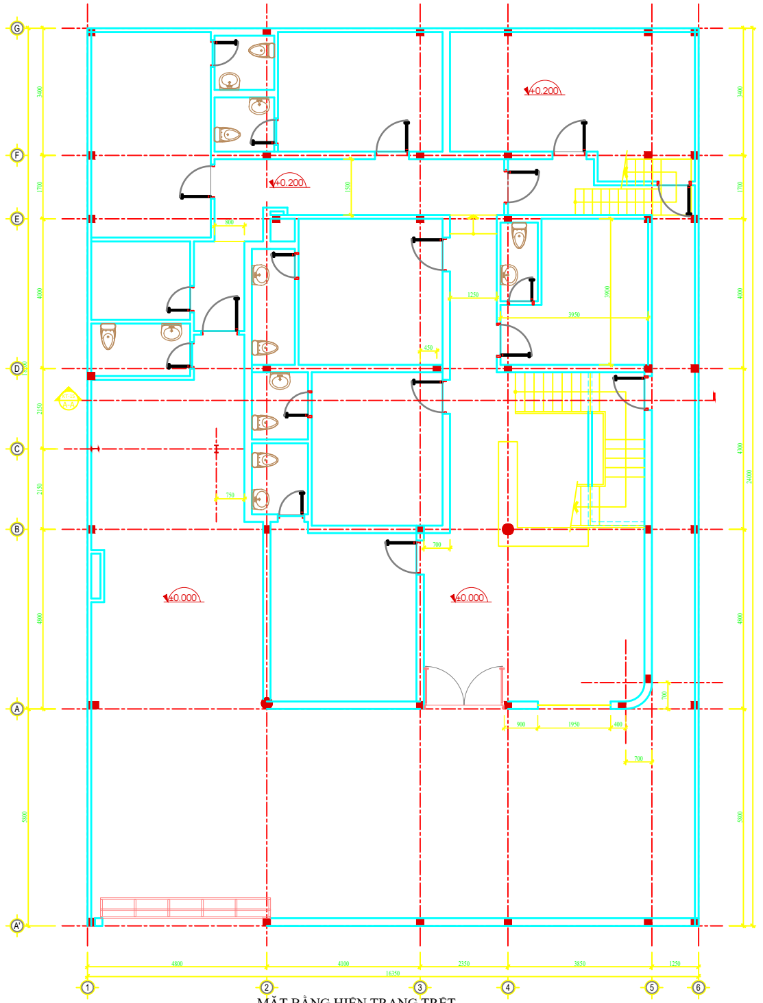
MẶT BẰNG HIỆN TRẠNG TRỆT TL: 1/100
