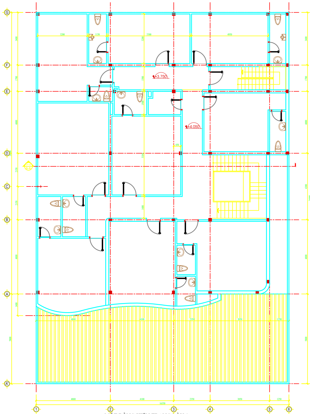
MẶT BẰNG HIỆN TRẠNG LẦU 1
