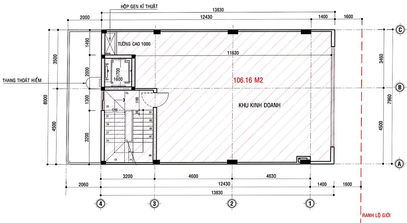
MẶT BẰNG LẦU 1
