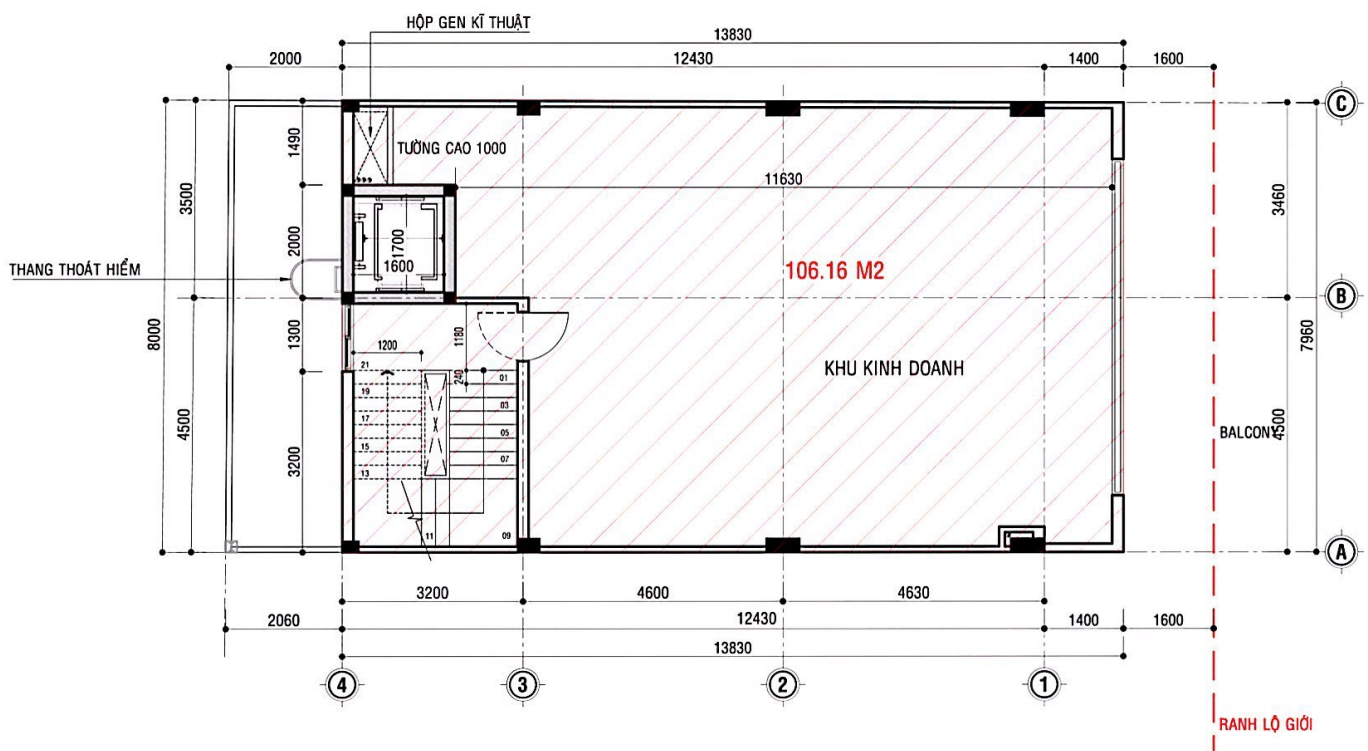
MẶT BẰNG LẦU 2
