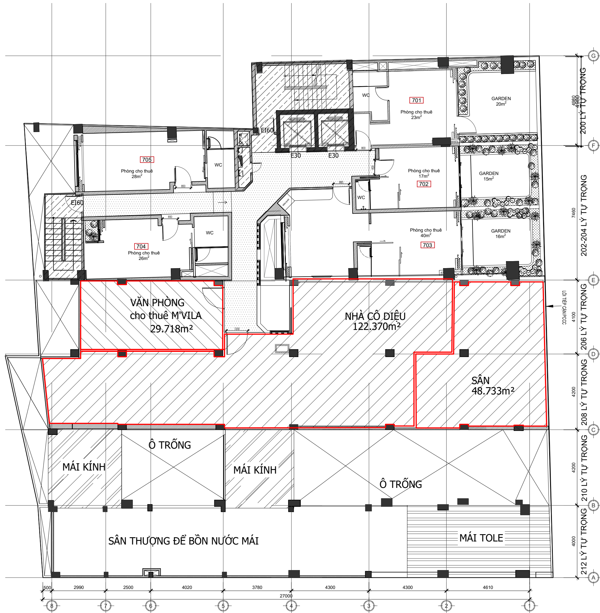
MẶT BẰNG TẦNG 7
