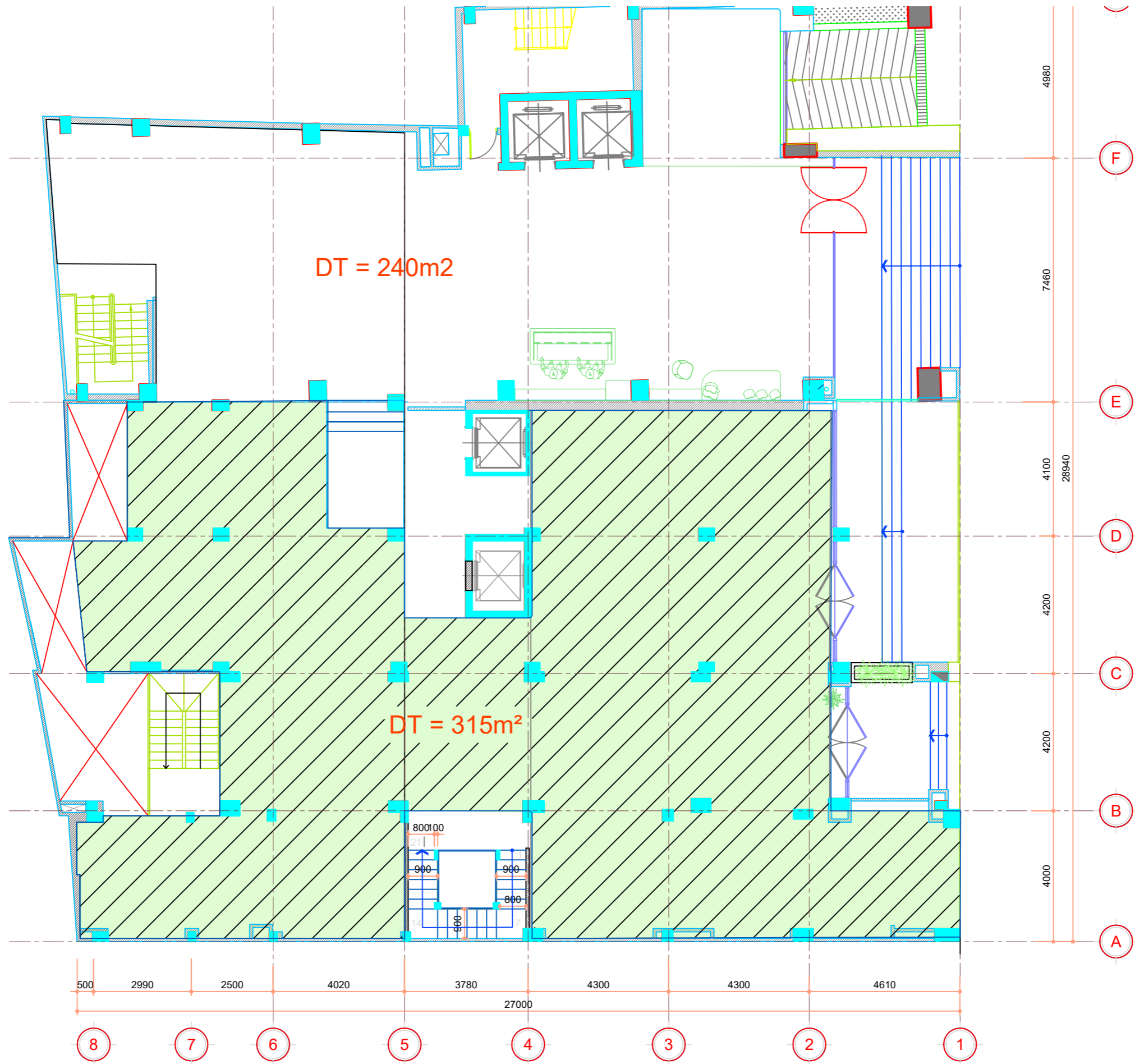
MẶT BẰNG BỐ TRÍ TẦNG TRỆT
