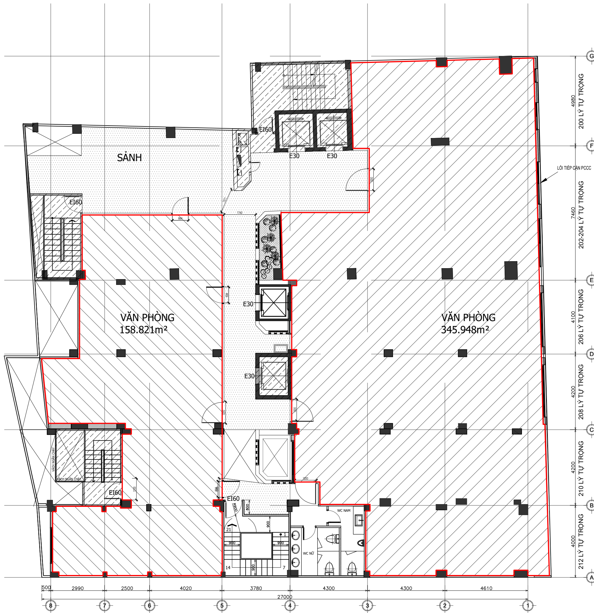
MẶT BẰNG TẦNG 2
