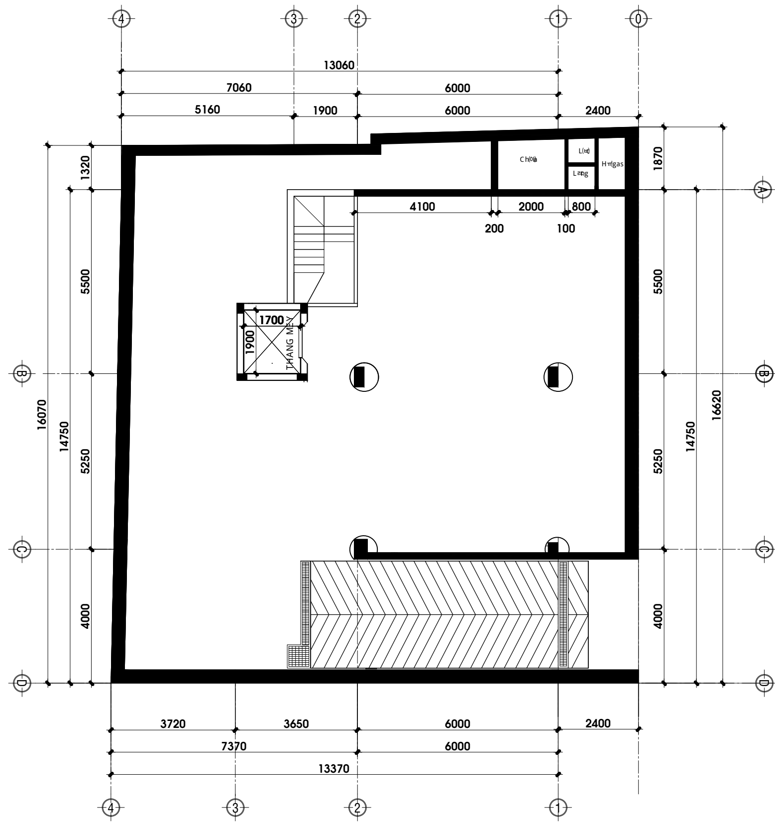
MẶT BẰNG T-NG H-M TL : 1%100
