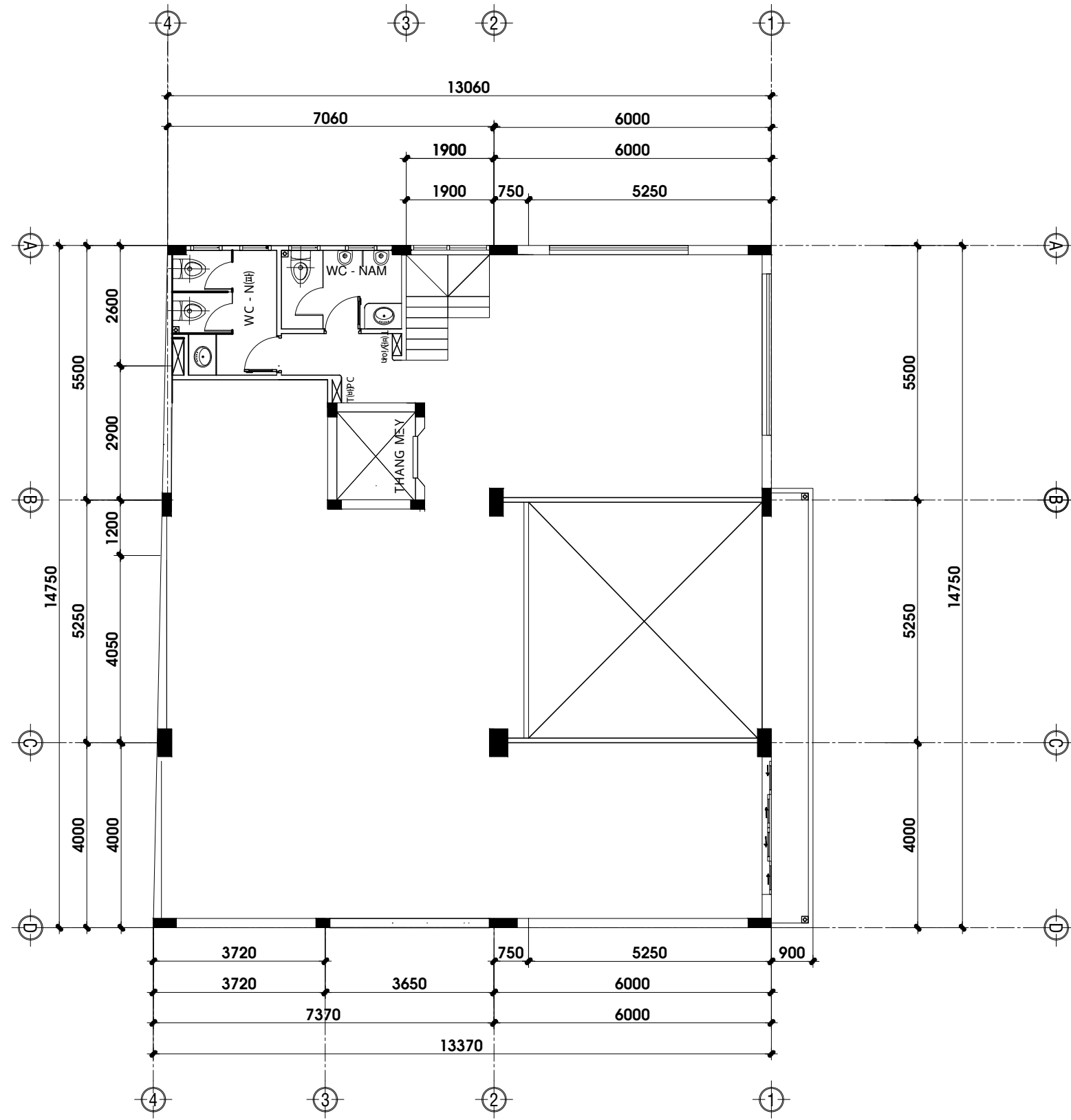
M ẦNG B ẦNG T ẦNG L (K ẦNG) TL : 1%100
