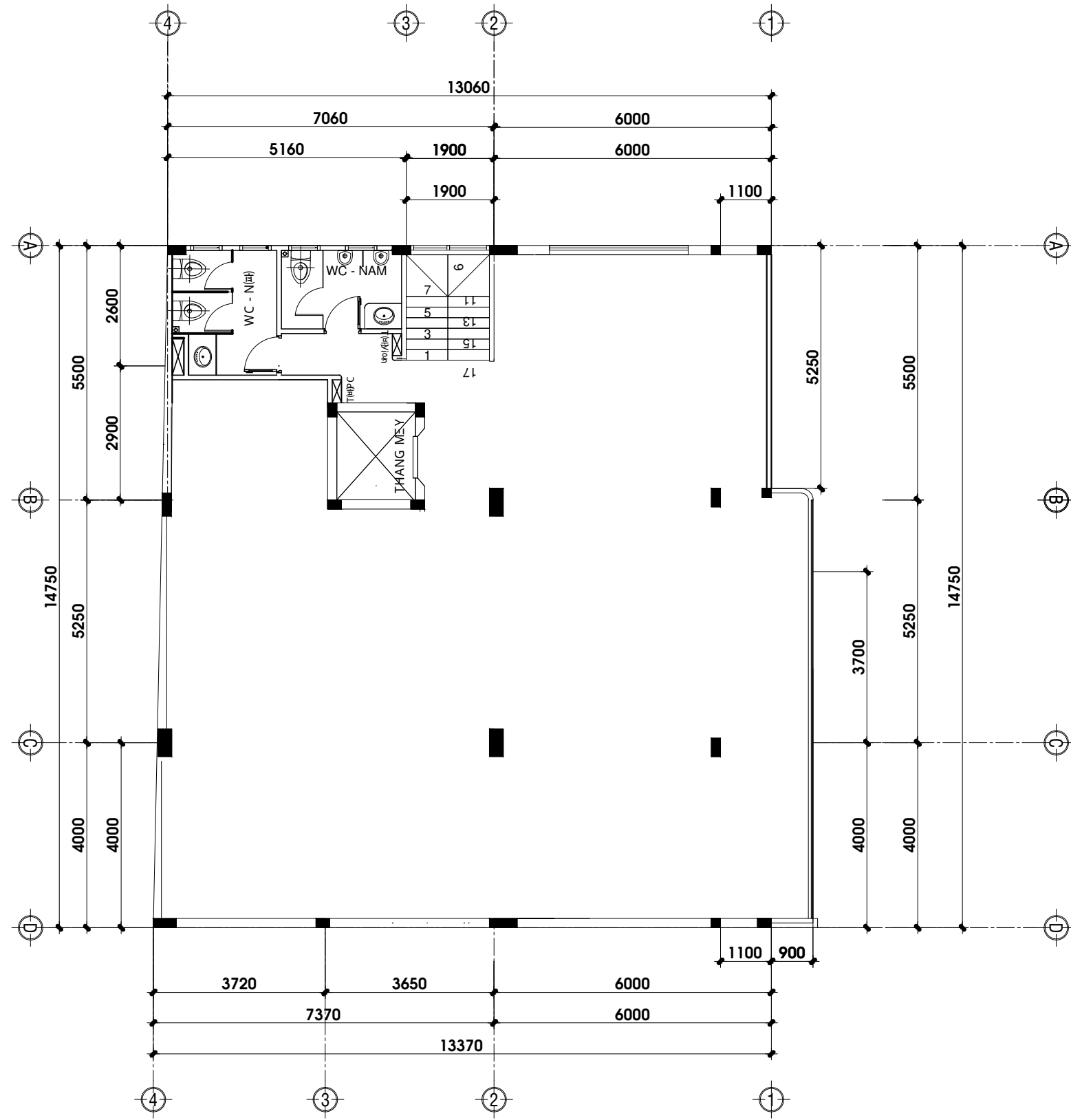
MẶT BẰNG L-03 TL: 1%100
