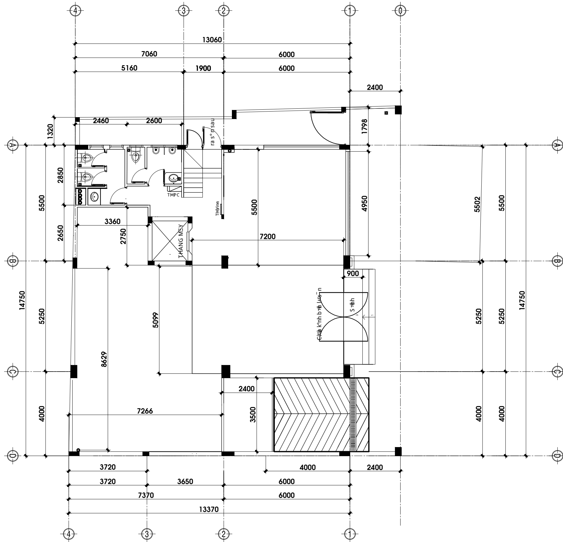
MẶT BẰNG T-NG TR Ơ T L : 1%100
